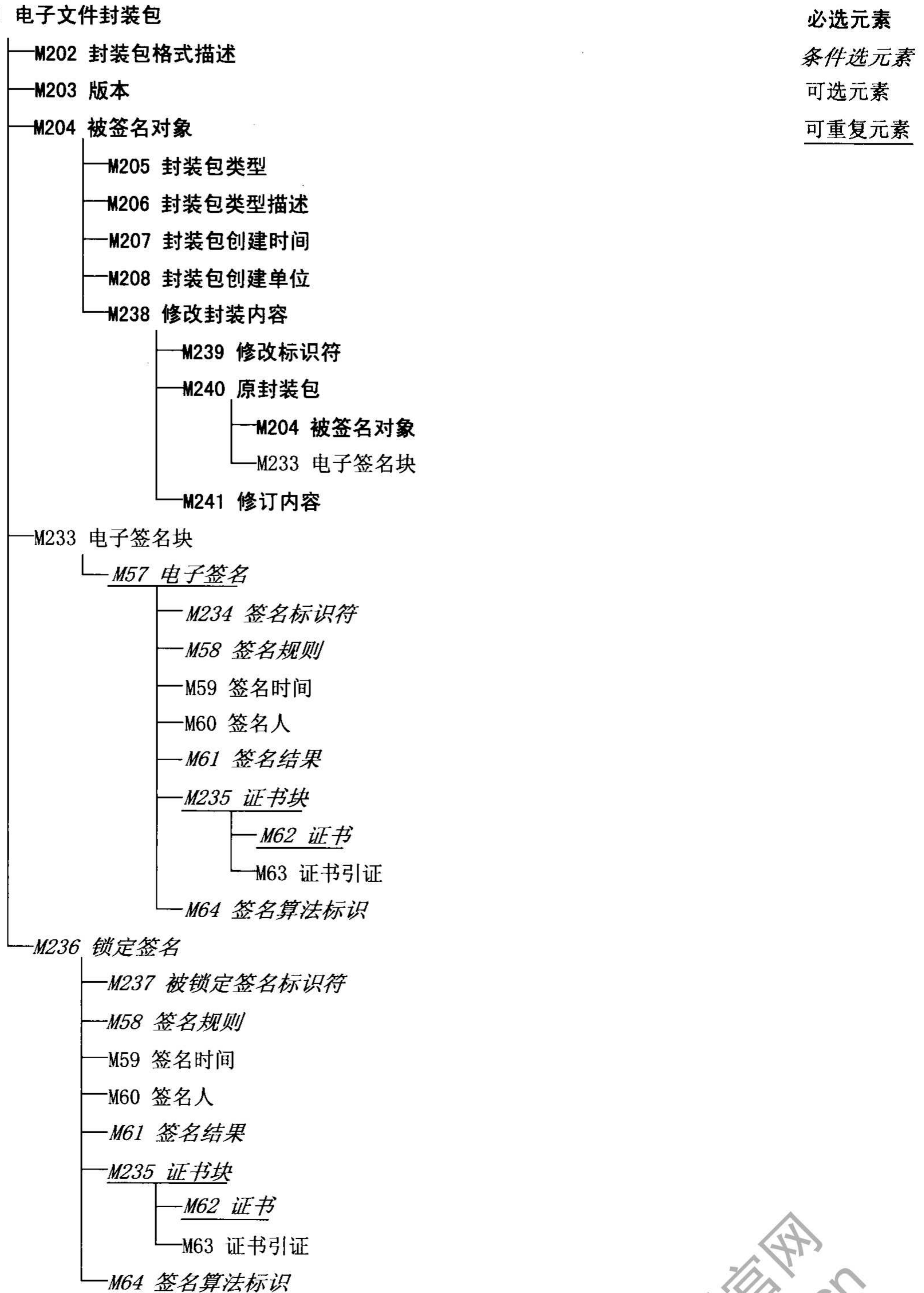
图A.2 修改型封装包树型结构图
